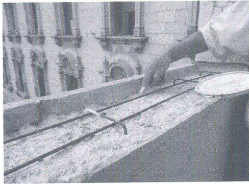
Fijación de los refuerzos de acero
