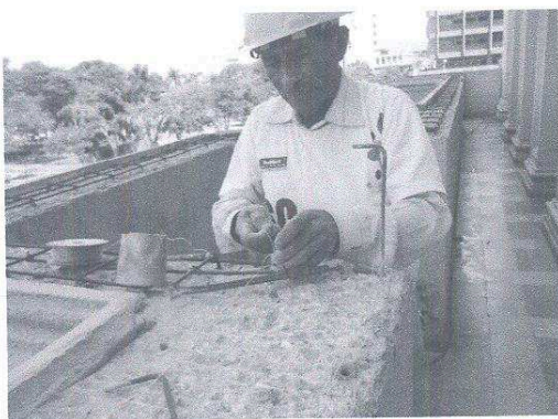
Colocando los refuerzo de acero con SIKA DUR 31 en el Pasamano
