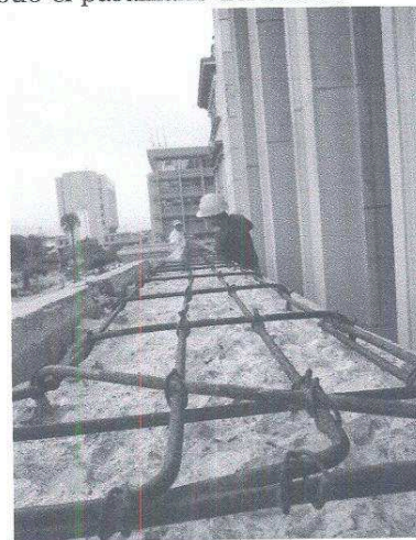
Colocación de los Refuerzos a lo largo de todo el pasamano del balcón
