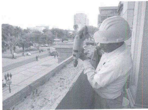
Barrenando para colocar los nuevos refuerzos de acero que se colocarán en el pasamano para volver a efectuar las integraciones necesarias
