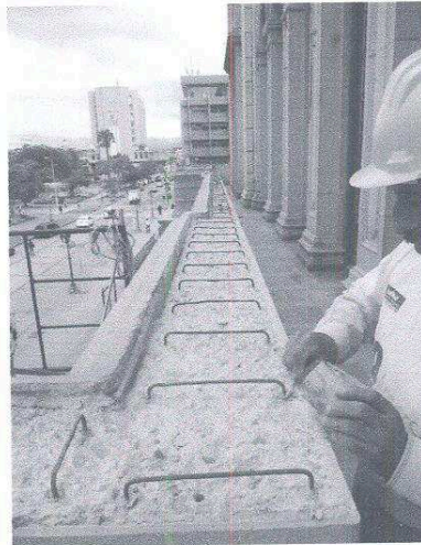
Colocando los hilos para colocar los refuerzos de acero y momentos en que se efectúa la colocación de los mismos
