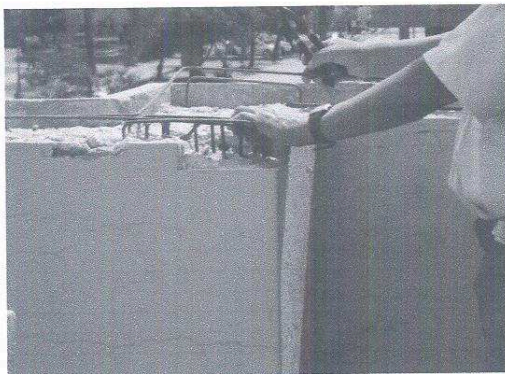
Colocación de los Refuerzos a lo largo de todo el pasamano del balcón
