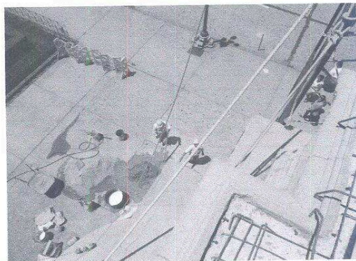
Formaleta finalizada y preparación de los elementos para la fundición
